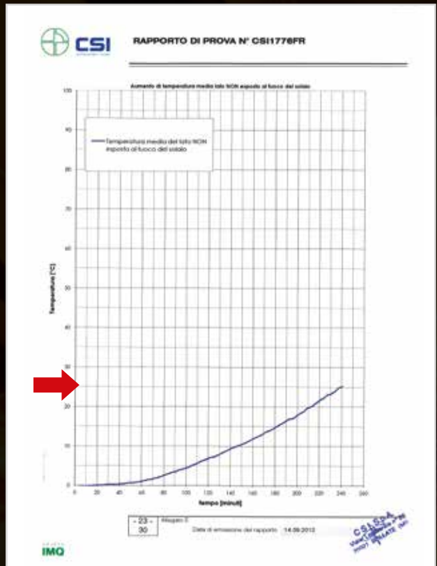
Temperatura de 25 °C, medida en el extradós de la losa, después de 240 minutos de exposición al fuego con temperaturas, del lado de la llama, de 1.100 °C
