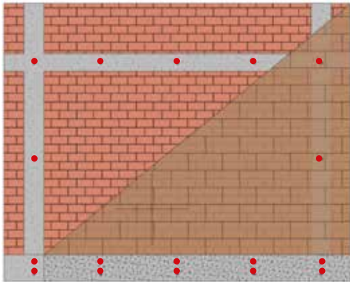
Colocación de conectores en las vigas de borde y rellenos
