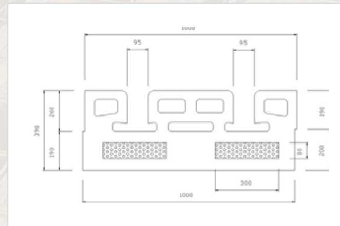
Bovedilla ISOTEX S39/S49 en madera cemento para cubiertas, garajes y locales no calefactados (bodegas, garages ecc.)
