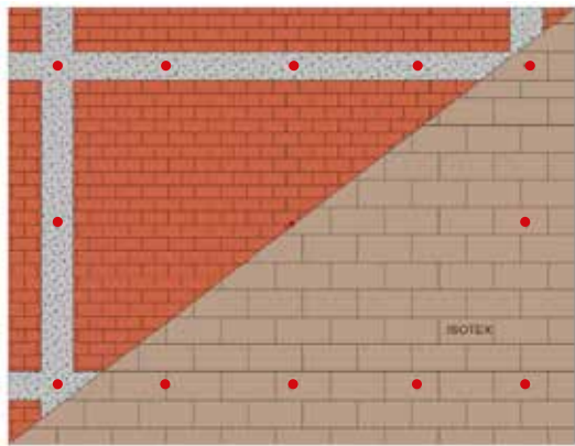
Colocación de conectores en las vigas de cimentación
